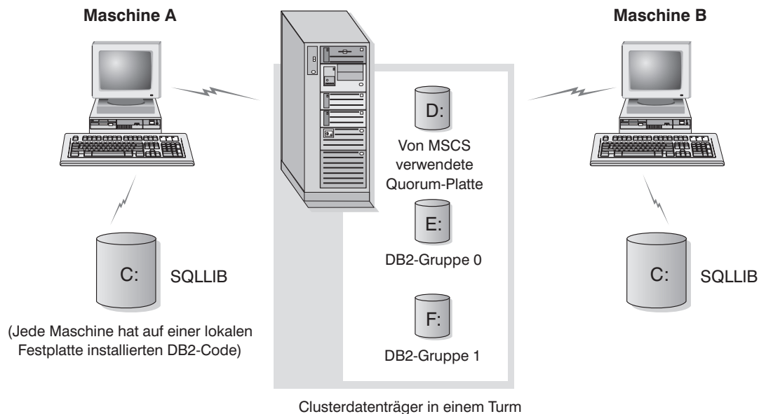
Abbildung 3. Beispielkonfiguration für Failover Clustering
